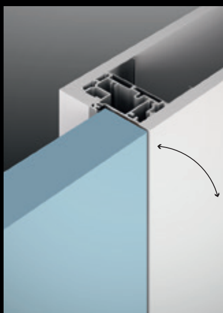
Pull Plain frame on plasterboard Stipite Plain a tirare su cartongesso Cadre Plain à tirer sur placoplâtre
